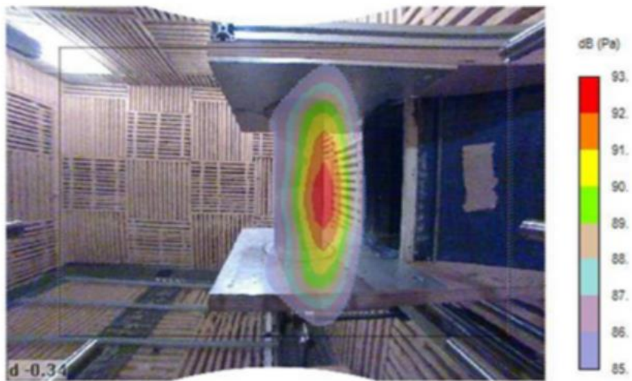
Atelier localisation de sources en écoulement : démonstration en soufflerie sur le site de l'Ecole Centrale.
